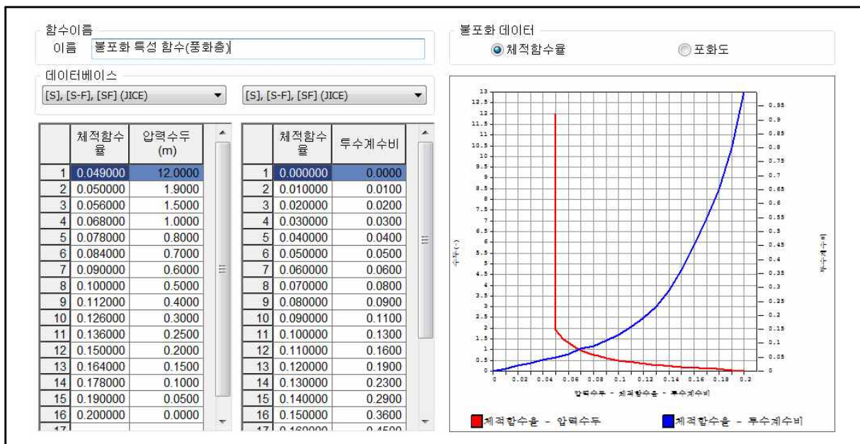
【그림 52.15】 압력수두-체적함수율(포화도)-투수계수비 함수
